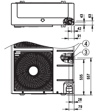
Przyłącza chłodnicze
